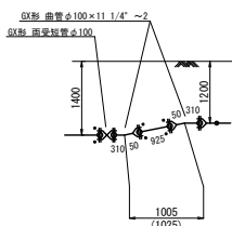
B断面詳細図
