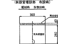
②市道As舗装部
