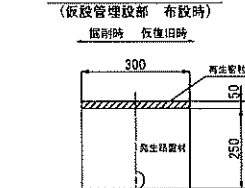
①市道As舗装部
