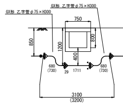
E断面詳細図
