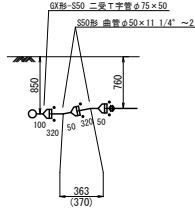
D断面詳細図
