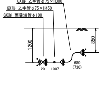
C断面詳細図
