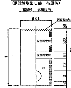
①市道As舗装部
