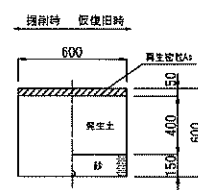
宅地内Co舗装部
