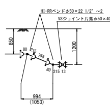
F断面詳細図
