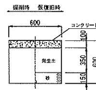
宅地内未舗装部
