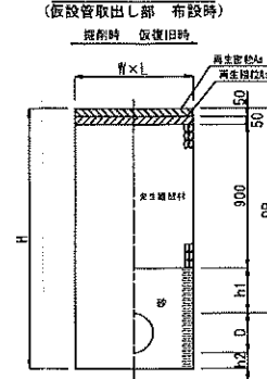
国道As舗装部
