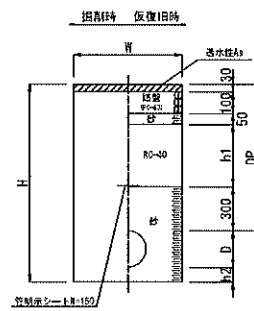
国道歩道As舗装部
