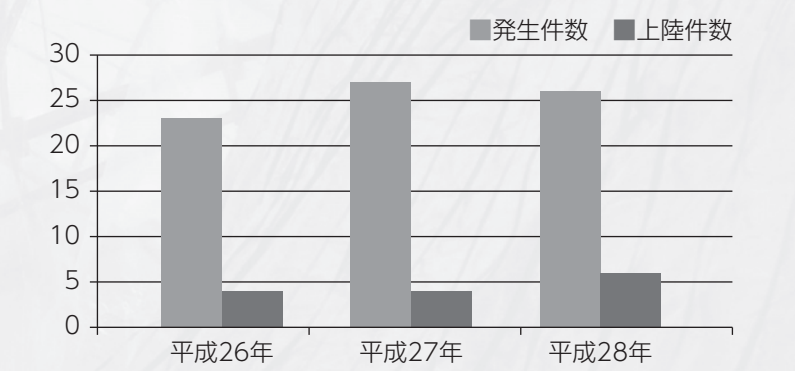
台風の発生件数と上陸件数
