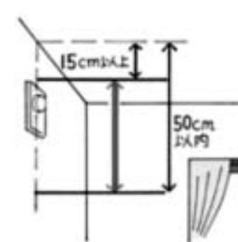
天井から15～50cm以内に住宅用火災警報器の中心がくるように取り付けます。
