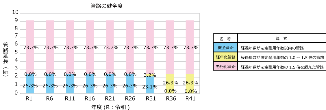
図 3-3-5 更新を実施しなかった場合の将来の健全度 (簡易水道事業)
