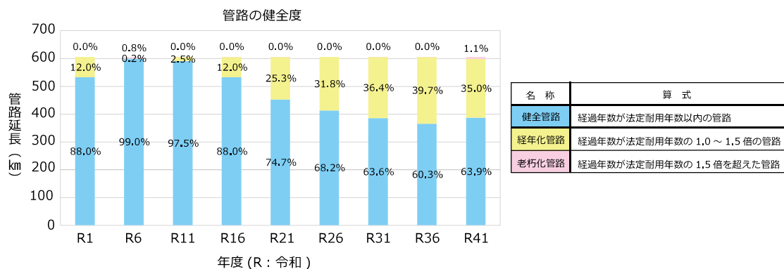
図 3-3-11 更新基準年数で更新した場合の将来の健全度（上水道事業）
