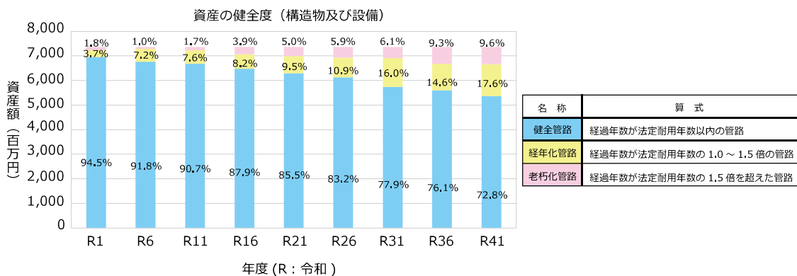
図 3-3-12 更新基準年数で更新した場合の将来の健全度（上水道事業）
