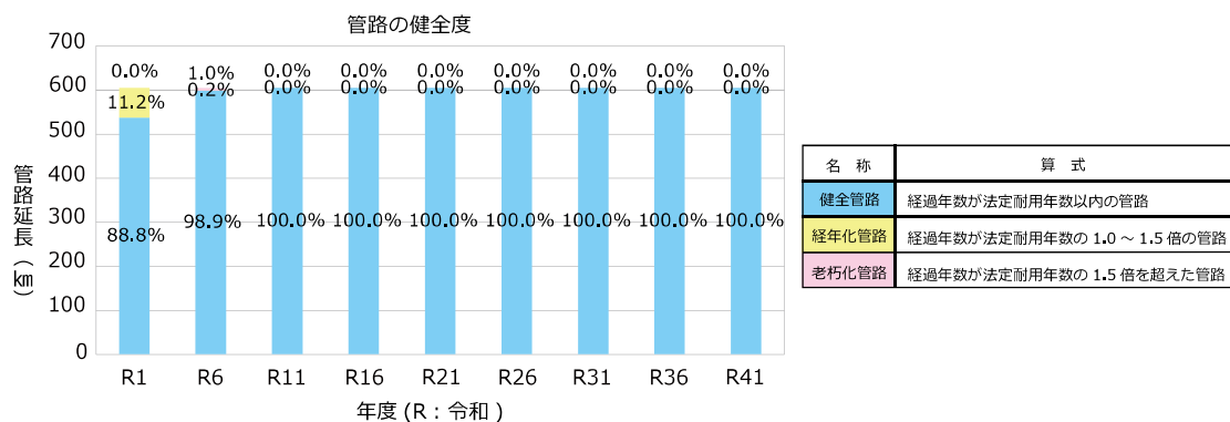
図3-3-7 法定耐用年数で更新した場合の将来の健全度（上水道事業）
